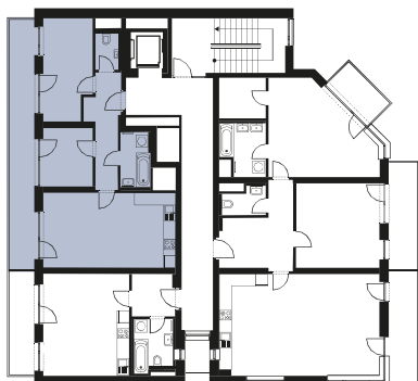
Celkový půdorys / total layout
