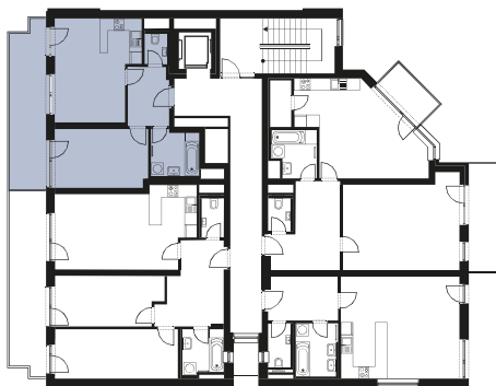
Celkový půdorys / total layout
